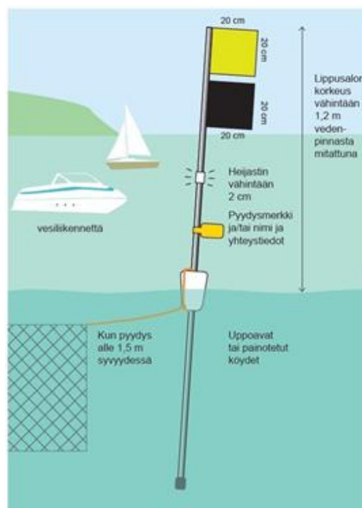
Kuva 2. Pintapyydys eli lähemmäksi kuin 1,5 metriä veden pintaa ulottuva pyydys, tulee vesiliikenteen käyttämillä alueilla merkitä kahdella päällekkäin kiinnitetyllä lipulla. (Piirros Anu Väitalo/KKL)
